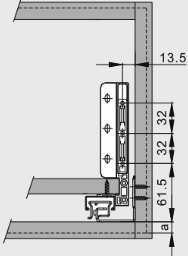
Монтаж передней панели
