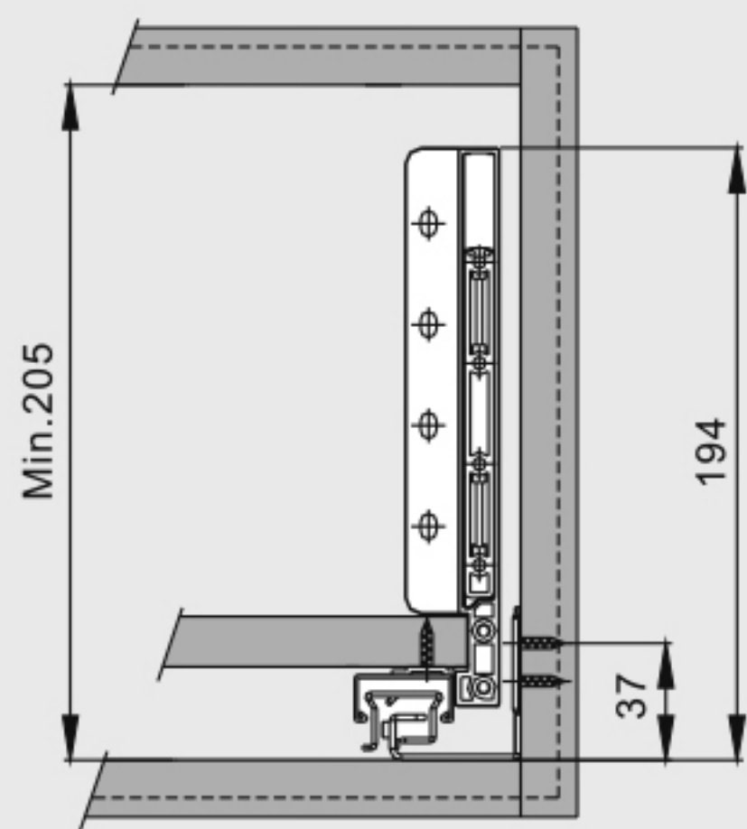
Внутренние размеры ящика
