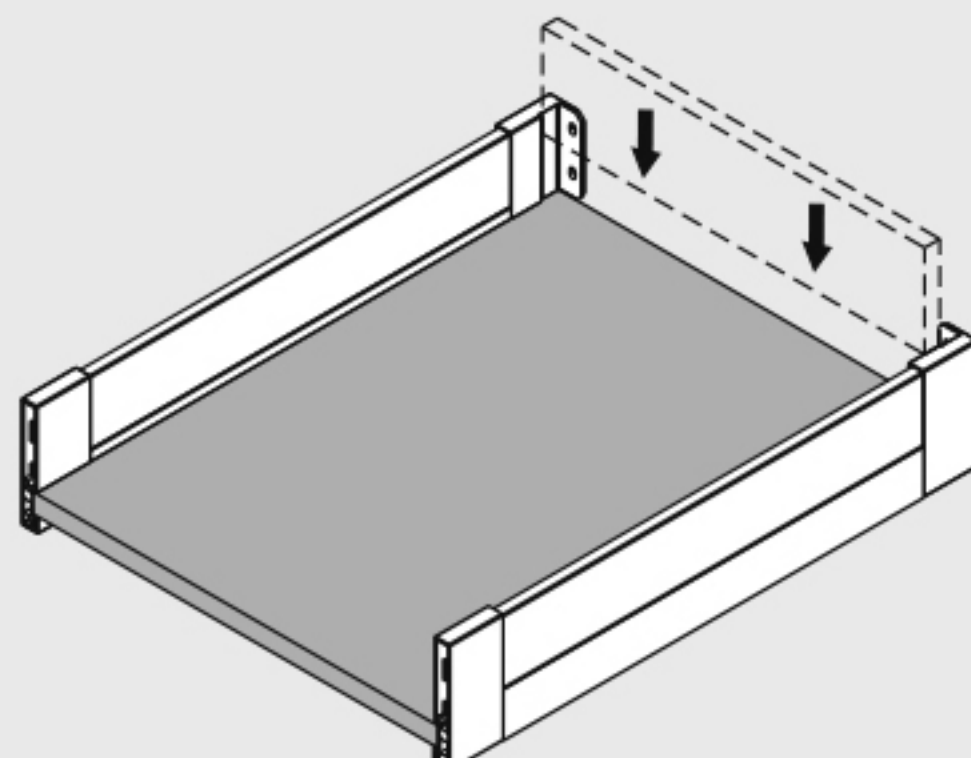
Монтаж задней панели
