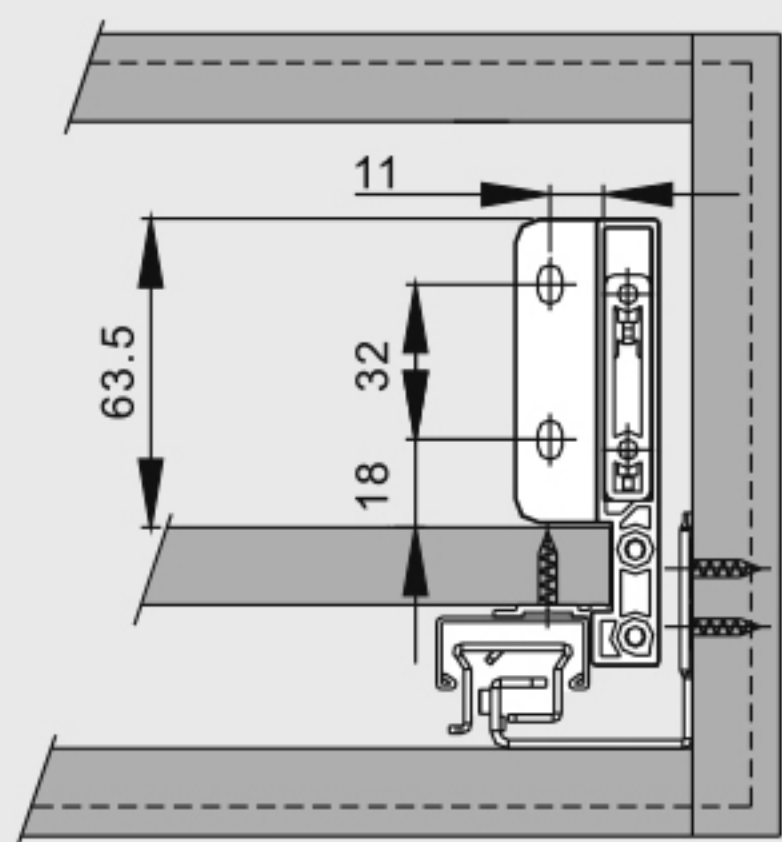
Монтаж задней панели
