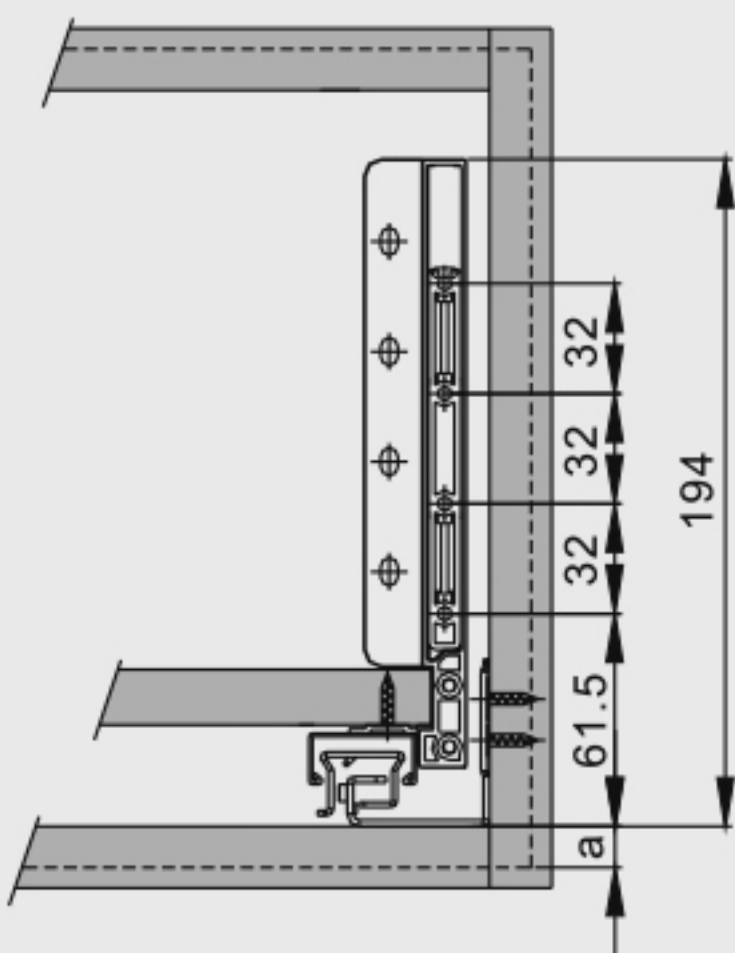
Монтаж передней панели
