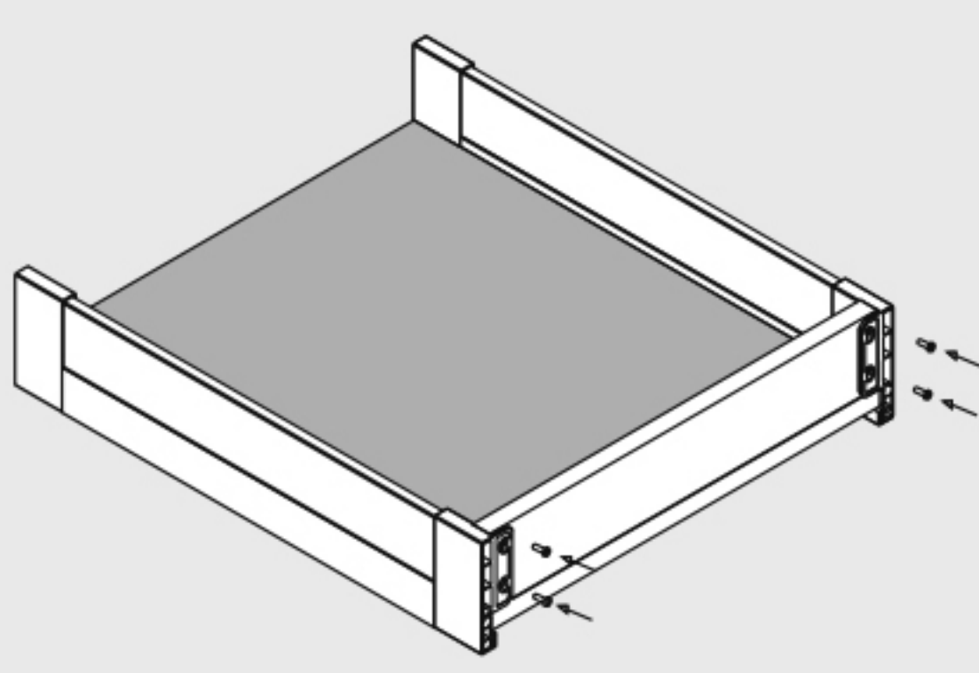
Монтаж задней панели
