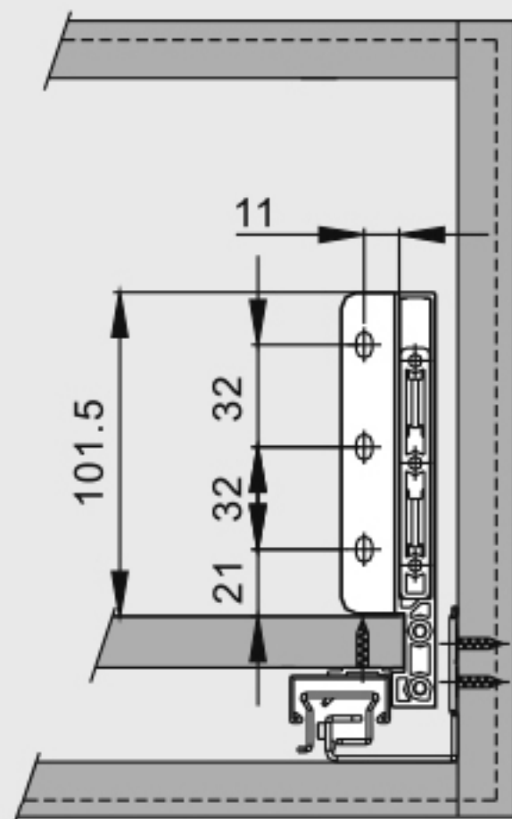
Монтаж задней панели
