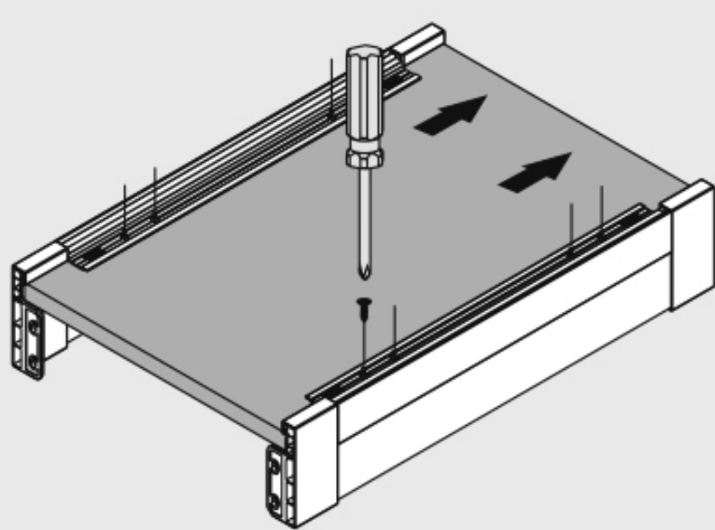
Монтаж дна ящика
