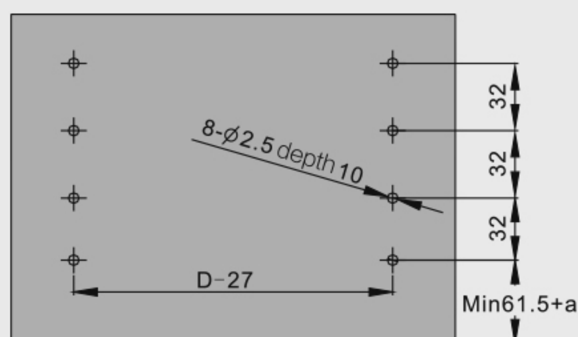
Монтаж передних фиксаторов
