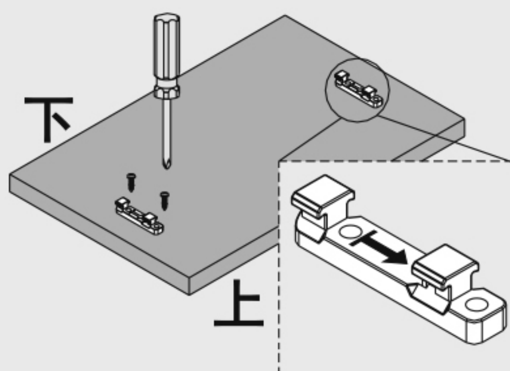
Монтаж переднего держателя
