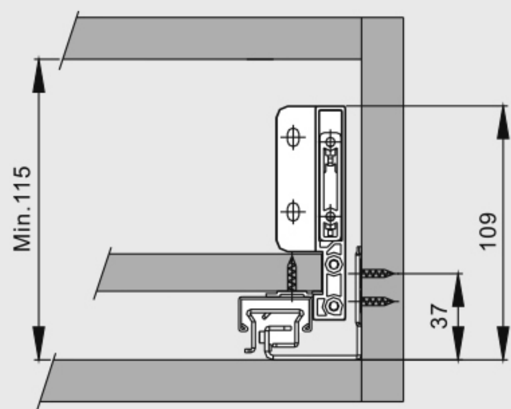
Внутренние размеры ящика
