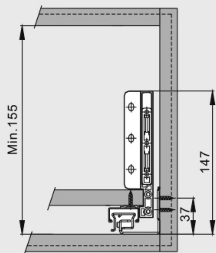
Внутренние размеры ящика
