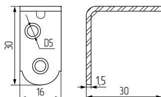
Уголок 30x30x16 ЦБ с ребром жесткости
