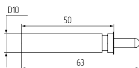
Газовый амортизатор Salice type
