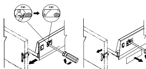
Демонтаж фасада
