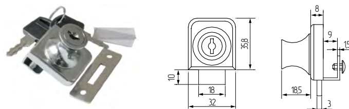
Замок 805.CR для 2 стеклянных дверей накладной, хром
