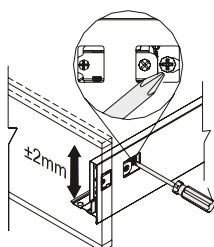
Регулировка фасада по высоте
