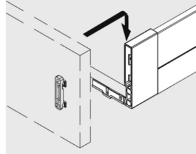
Крепление передней панели
