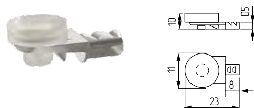
Полкодержатель для стеклянной полки 5x8 с амортизатором
