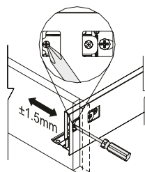
Регулировка фасада влево-вправо
