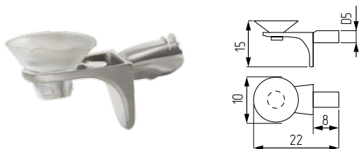
Полкодержатель Г-образный для стеклянной полки 5x8 с амортизатором
