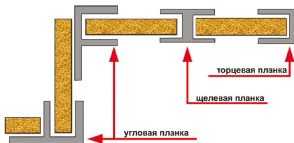
Планка торцевая для панелей 600 мм
