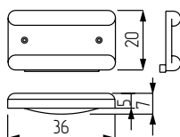
Подпятник с гвоздиком D-15 мм
