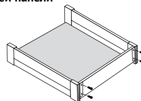
Монтаж задней панели
