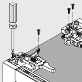
Монтаж фиксатора Clip-On
