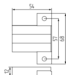
Держатель для газового амортизатора двух дверей
