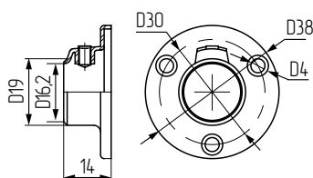
Фланец рейлинга D16 мм, стальной
