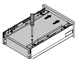
Сборка ящика на саморезы
