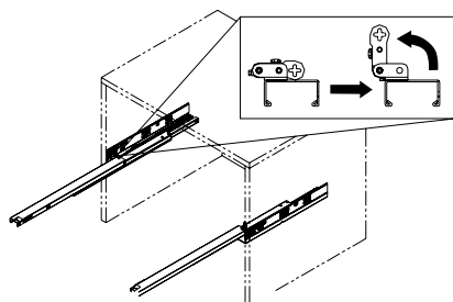
Установка направляющих
