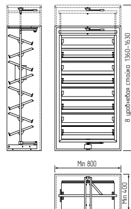
Схема артикула 10964
