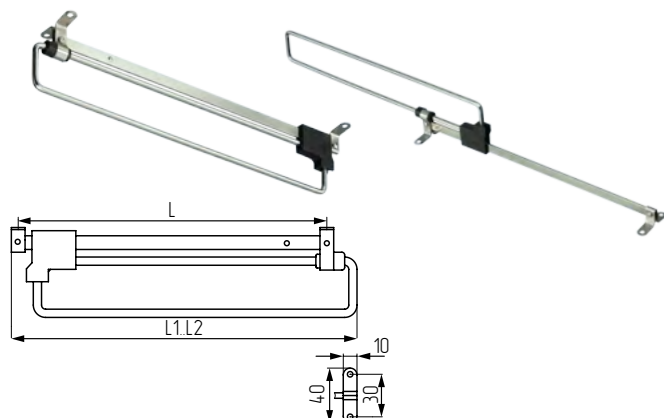
Штанга выдвижная, никель
