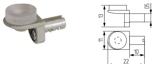
Полкодержатель 5x10 с амортизатором
