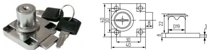
Замок 202.CR для шкафа-купе, Ø19x22, хром
