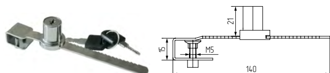
Замок 318 реечный для раздвижных стеклянных дверей, хром, полотно 140мм
