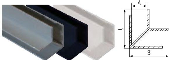
Планка угловая для панелей 600 мм (внутренний угол 90°)
