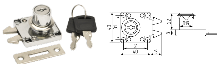
Замок 338.CR автомат Ø19x22, хром
