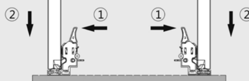
Отсоединение ящика
