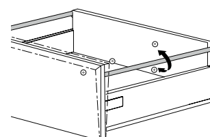
Регулировка рейлинга по глубине
