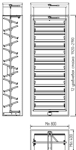
Схема артикула 10965
